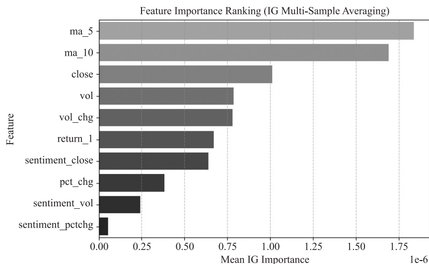
图8 多模态特征重要性排序
