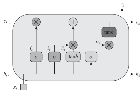
图4 单通道 LSTM 基本框架
